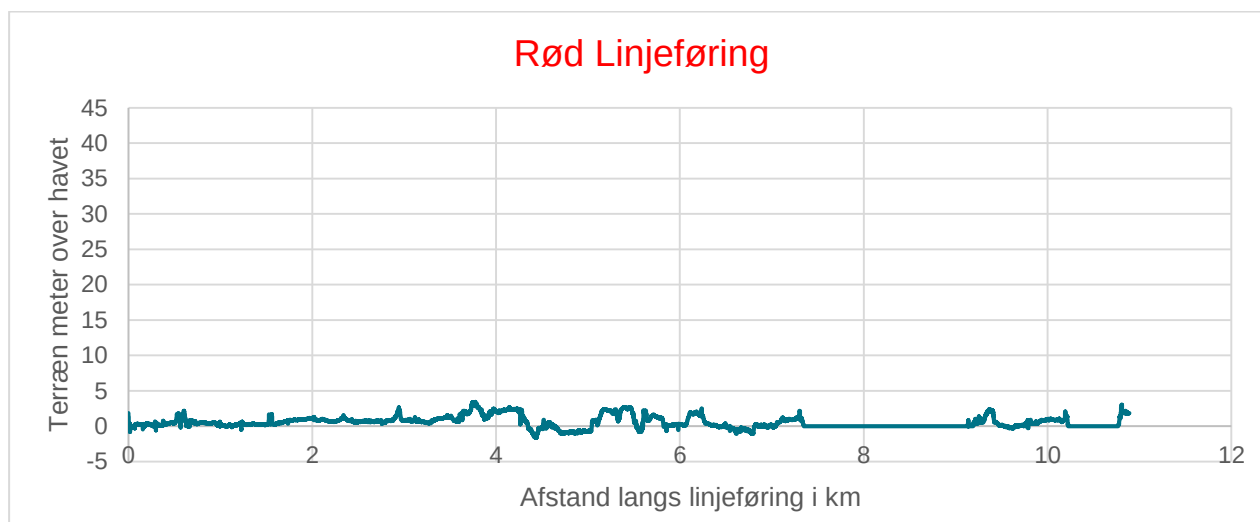
Figur 5: Terræn (meter over havet) langs grøn og rød linjeføring, idet "0 km" = startpunktet ved Lemvig (Danmarks Højdemodel 2019). Rød linjeføring har stort set samme terrænforhold som lilla linjeføring.
